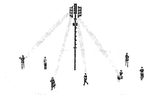
Antenne active 5G avec système d'émission et réception directionnel des signaux fréquences > 10 GHz
